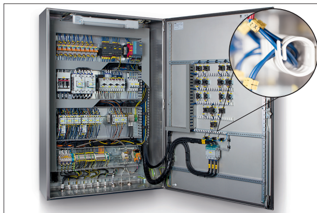
Heladuct flex pode ser instalado em ângulos acima de 90°.
