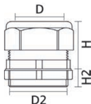
Prensa cabos.
